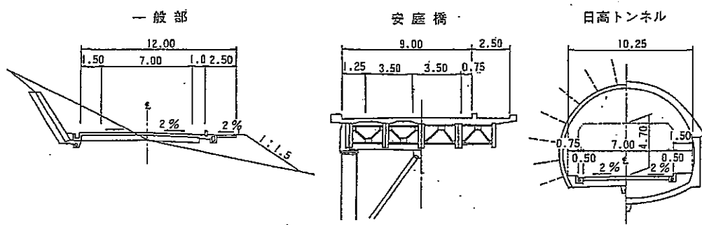
標準横断面
