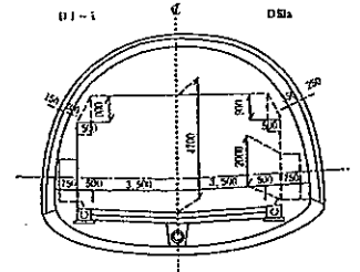
トンネル標準断面図
